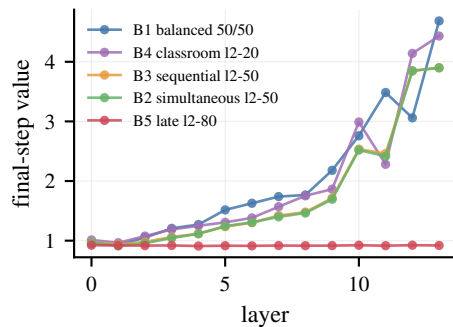
\|W_{OV}\|_F
