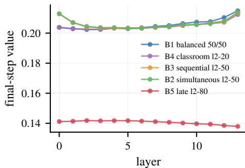
Hoyer( W_{\text{SwiGLU}} )
